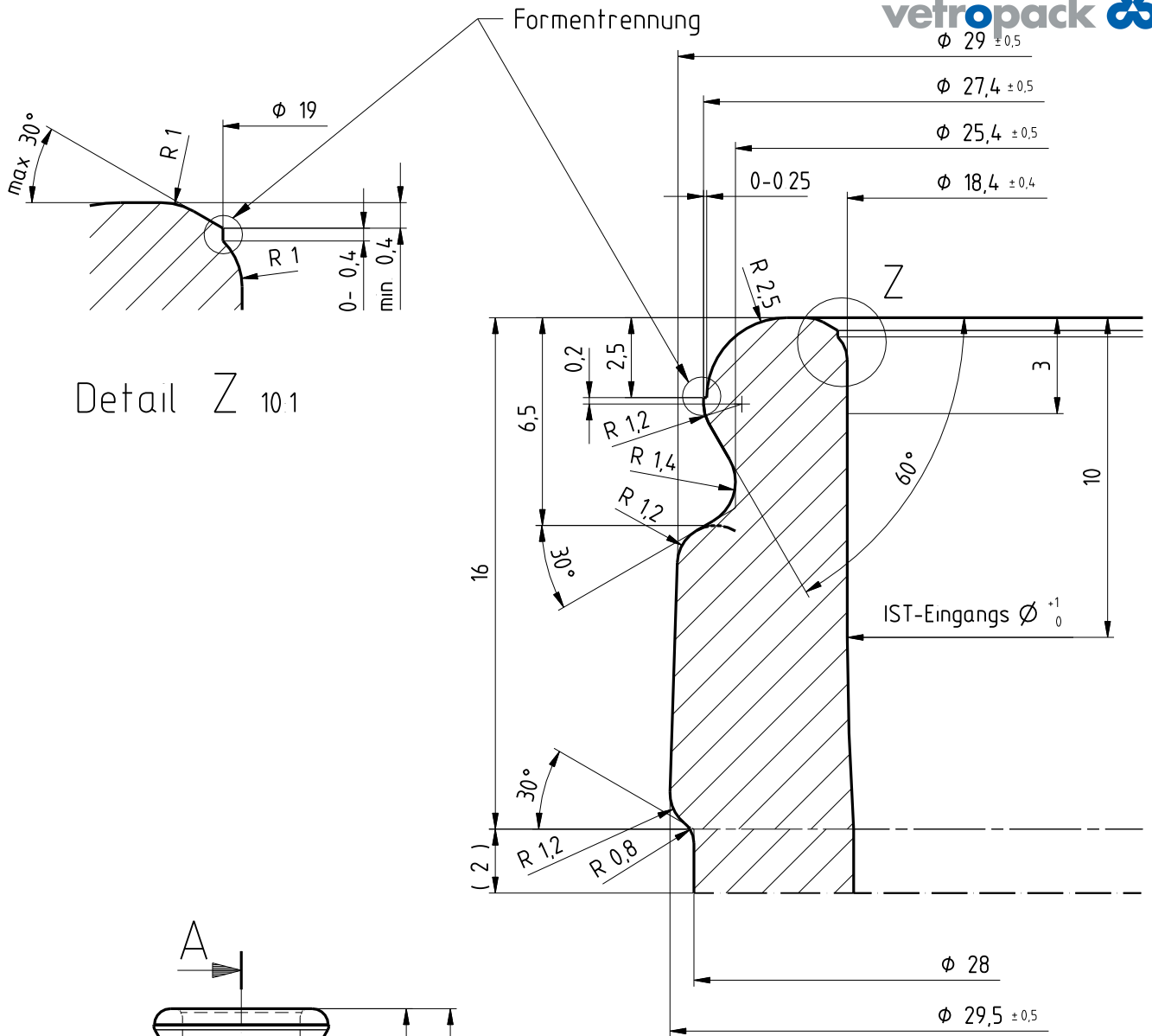
Schnitt A-A 51
